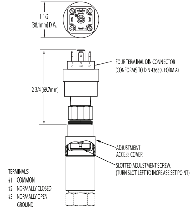
OPTION M515 DIN CONNECTOR
