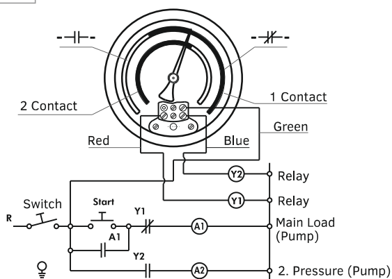
NONC
